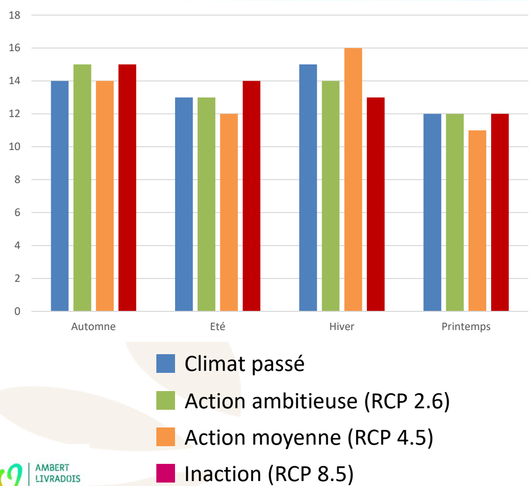
Nombre de jours de sécheresse par an
